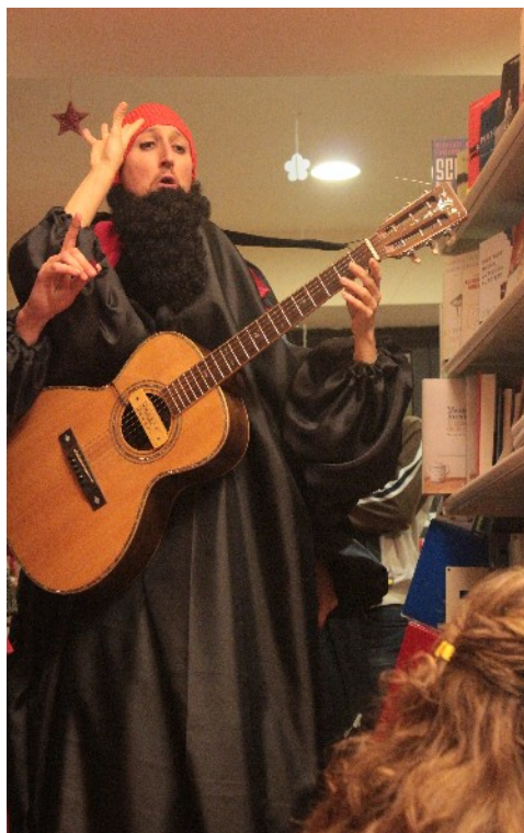
Encelado, il gigante a quattro braccia
